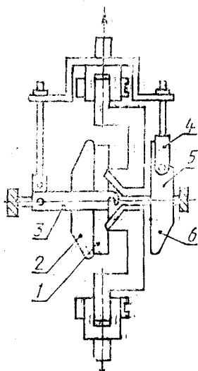
1 — образец; 2 — упорная планка; 3 — планка; 4 — захват; 5 — упор; 6 — траверса
